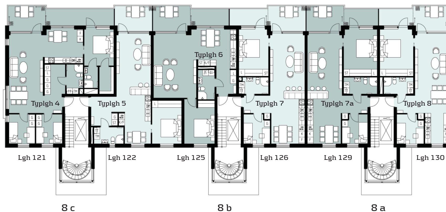
Översikt plan 4 Skala 1:200
